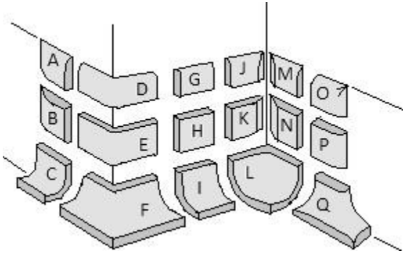
Vista explodida - Ladrilhos de acabamento em três fileiras
